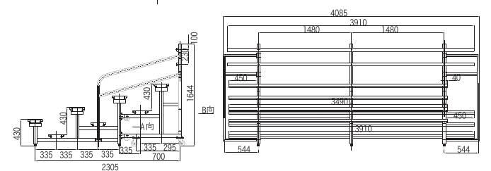
LP-4 四层看台 LP-4 Four-Row Bleacher Without Back 四层看台 4085X2450X1640 平板铝合金座板 240X60X3490 铝合金踏板 240X60X3910
