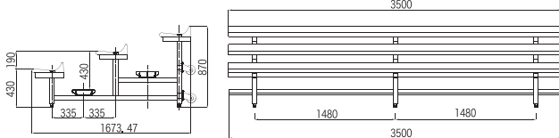
LD-3 三层看台 LD-3 Three-Row Bleacher With Low Back 三层看台 3500X1670X870 低靠铝合金座板 330X110X3500 铝合金踏板 240X60X4000
