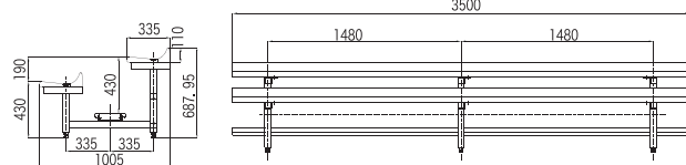
LD-2 二层看台 LD-2 Two-Row Bleacher With Low Back 二层看台 3500X1005X69 铝合金座板 330X110X3500 铝合金踏板 240X60X400
