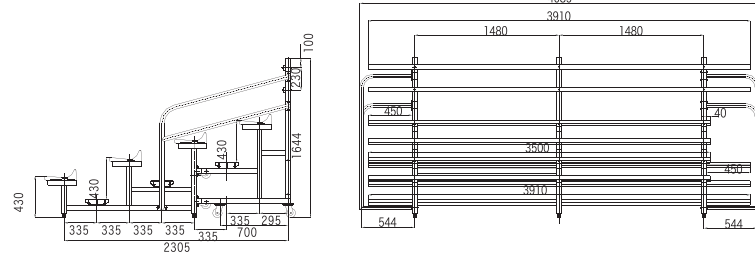
LD-4 四层看台 LD-4 Four-Row Bleacher With Low Back 四层看台 3500X1670X2540 低靠铝合金座板 330X110X3500 铝合金踏板 240X60X3910
